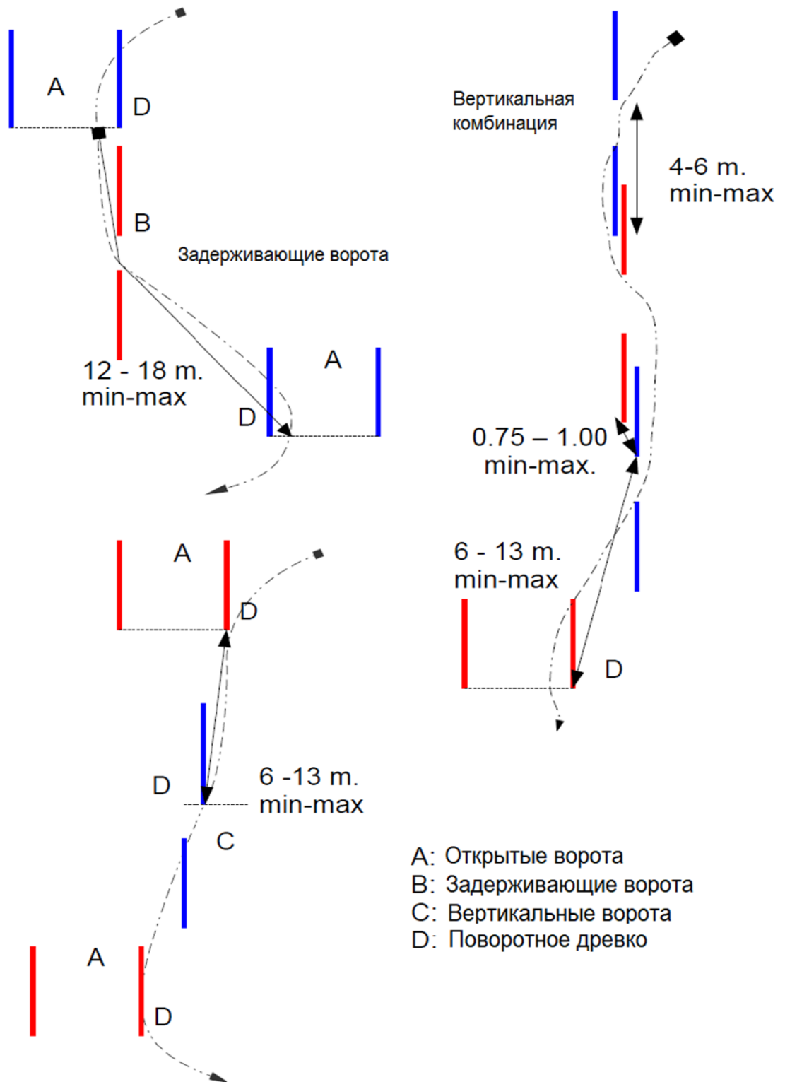
Рисунок 2. Схема постановки трассы слалома.
